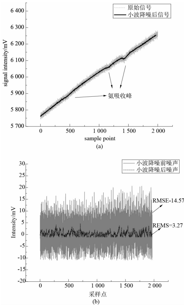
图2 (a)小波降噪前后的信号,(b)小波降噪前后的均方根误差分析
