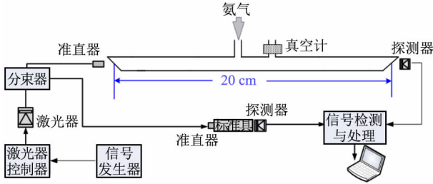
图1 光谱测量实验平台
