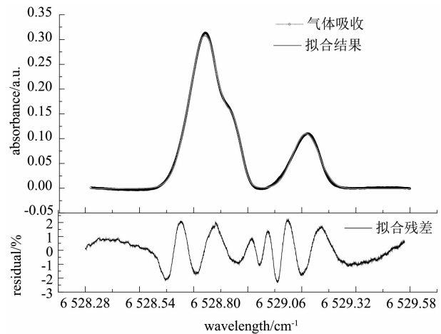
图3 Voigt 线型拟合结果分析 Fig.3 Analysis of multi-line Voigt line profile fitting
