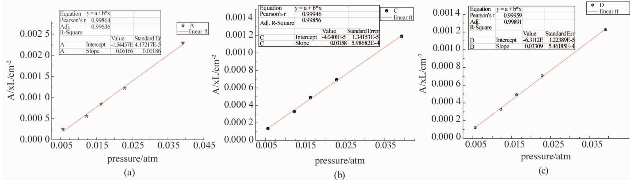
图6 (a) 6528.76 cm -1 处的吸收线强计算结果,(b) 6528.8998 cm -1 处的吸收线强计算结果,(c) 6529.1901 cm -1 处的吸收线强计算结果
