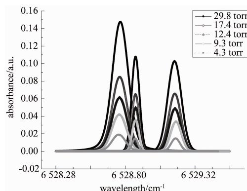
图 5 混叠吸收谱线分离 Fig. 5 Multi-line separation
